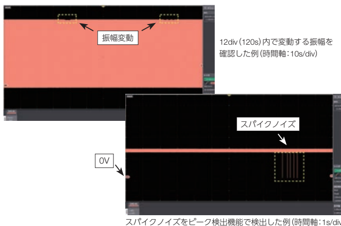
スパイクノイズをピーク検出機能で検出した例(時間軸:1s/div)
