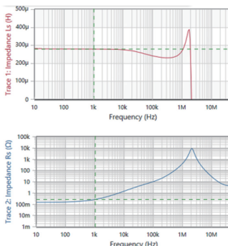
Ls・Rs-周波数
