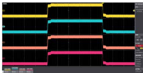
16384 回波形補足結果
