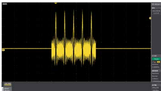
ランダム性ノイズが多く含まれるパルス波形
