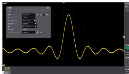
高分解能モードでノイズを低減した波形
