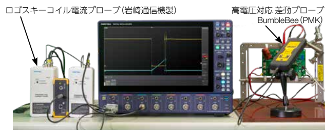
GaNデバイス評価基板のスイッチング電圧・電流 測定例
