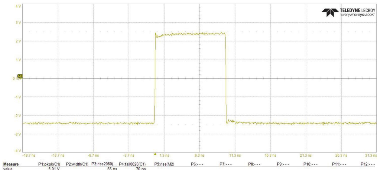
Rider FastEdge™ 立上り／立下り時間 70ps, 5Vpp
