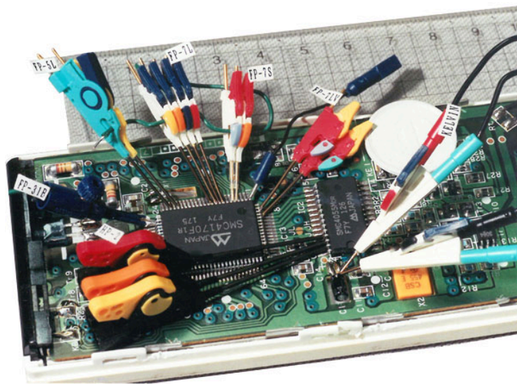
メカノクリップ各種 接続例
